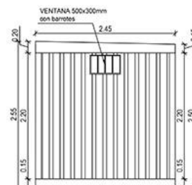
VISTA LATERAL DERECHA Esc: 1/40
