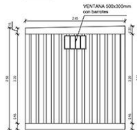
VISTA LATERAL IZQUERDA Esc: 1/40
