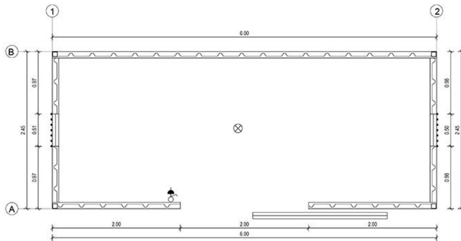
PLANTA DE ARQUITECTURA Esc: 1/25
