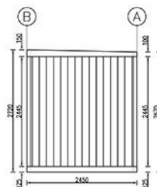
ELEVACION EJE 4 ESC. 1:50
