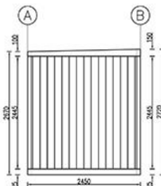
ELEVACION EJE 1 ESC. 1:50
