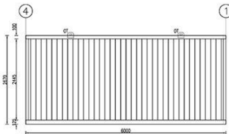
ELEVACION EJE A ESC. 1:50
