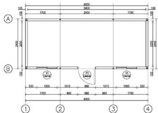
PLANTA DE ARQUITECTURA ESC. 1:50
